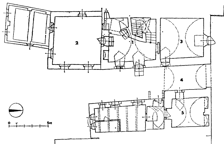
Obr. 2. Úštěk čp. 18 (okres Litoměřice), půdorys přízemí předměstského, převážně pozdně gotického domu. Nahoře obytné stavení, dole křídlo, vzniklé přístavbou k někdejší sýpce. 1 — síň, 2 — světnice, 3 — komora, 4 — průjezd, 5 — přízemí někdejší sýpky. Podle zaměření SÚPPOP v Praze z roku 1954.
