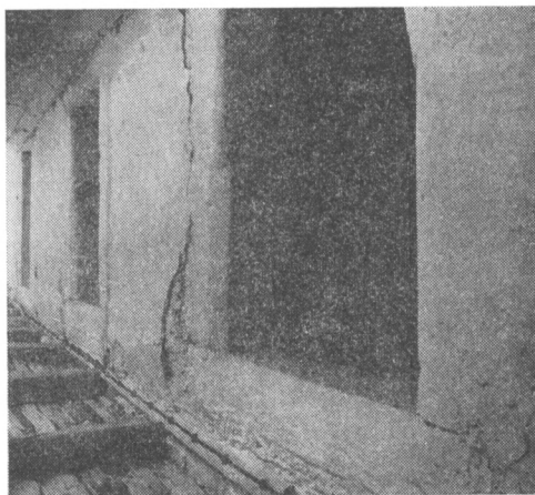
Obr. 1. Soběnlce čp. 6 (okres Litoměřice), pozdně gotické portály ze 2. poloviny 16. století na pavlači v patře sýpky. Foto J. Škabrada, 1977.
