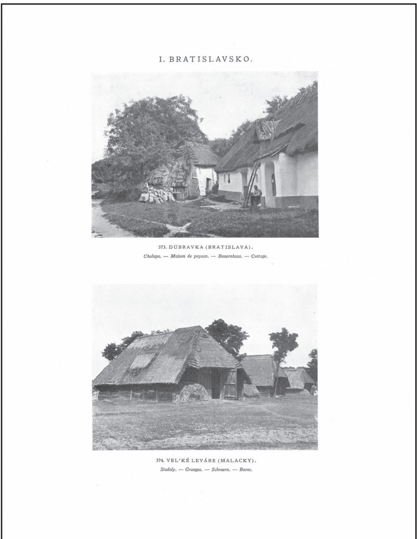
374 Velké Leváře (Malacky). Podélně průjezdné stodoly, které se stavěly v rozsáhlé nížinné oblasti pod karpatským obloukem na rozhraní střední a východní Evropy, ve starším dřevěném provedení - s lehkou rámovou konstrukcí a doškovou krytinou.
