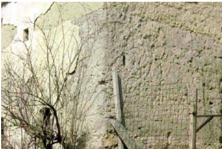
hliněné konstrukce * 96 - Popice - vrstvená konstrukce stěny lisovny * 97 - Hnanice - vrstvená konstrukce stěny lisovny (nakládané nebo z válků dusaných do bednění) s nadstavbou z nepálených cihel * 98 - Šatov - nakládaná stěna lisovny * 99 - Hnanice - sklep hloubený v rostlé hlině
