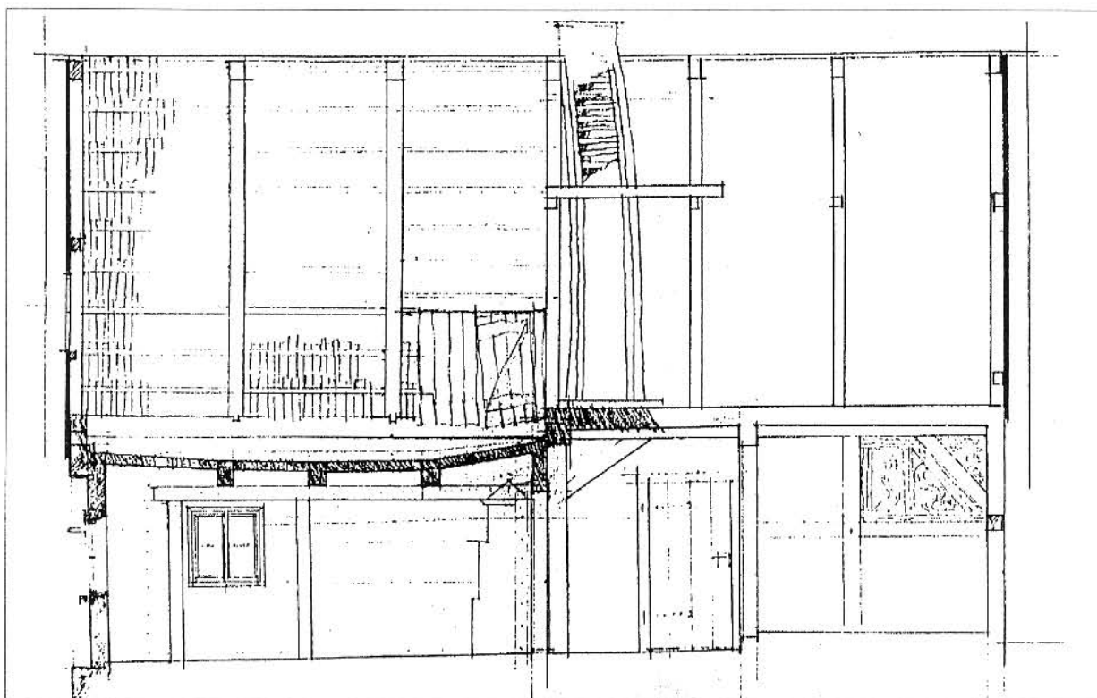
Šluknov č.p. 310 - podélný řez
