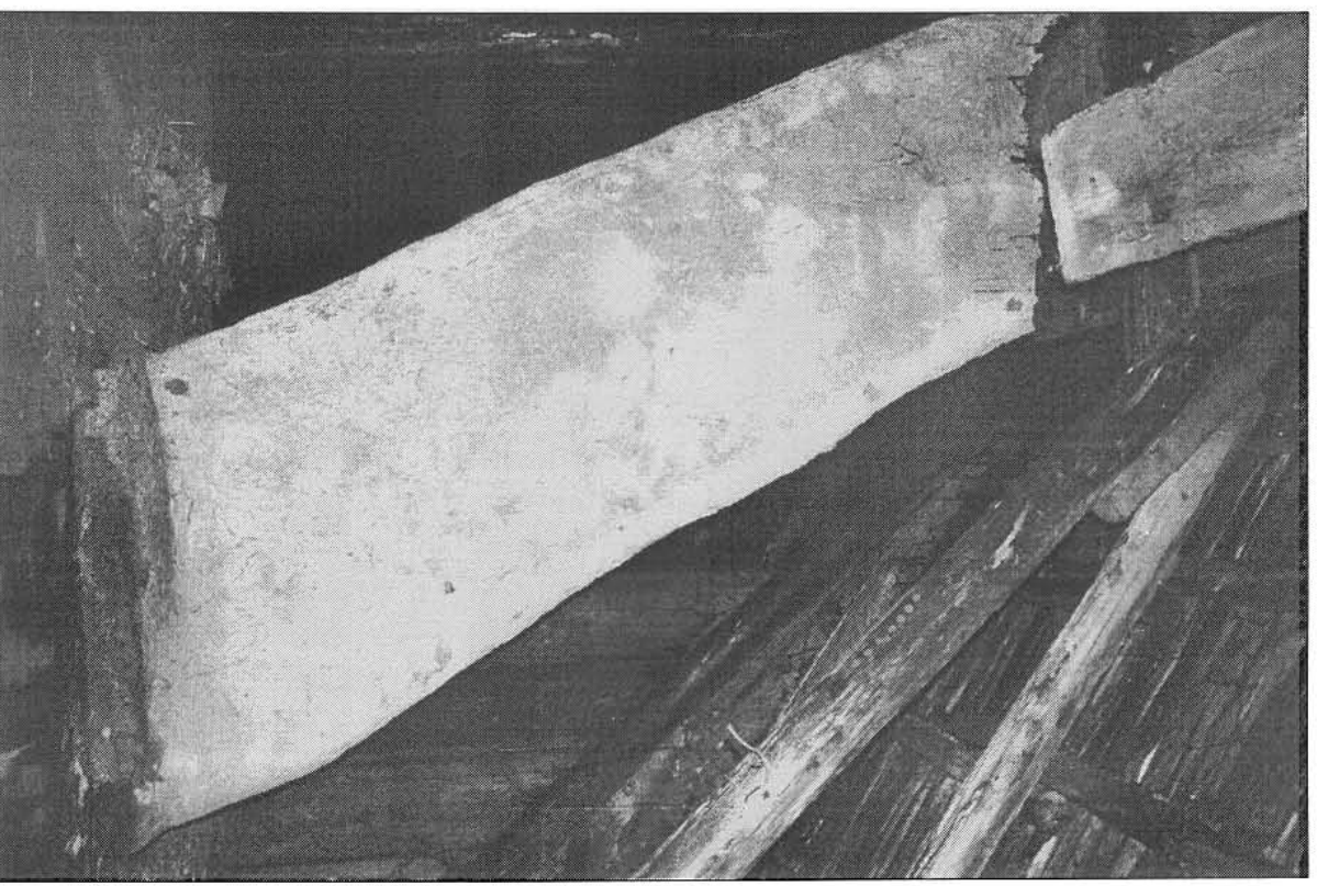
Šluknov č.p. 310 těleso dřevohliněného komína v podkrovní
