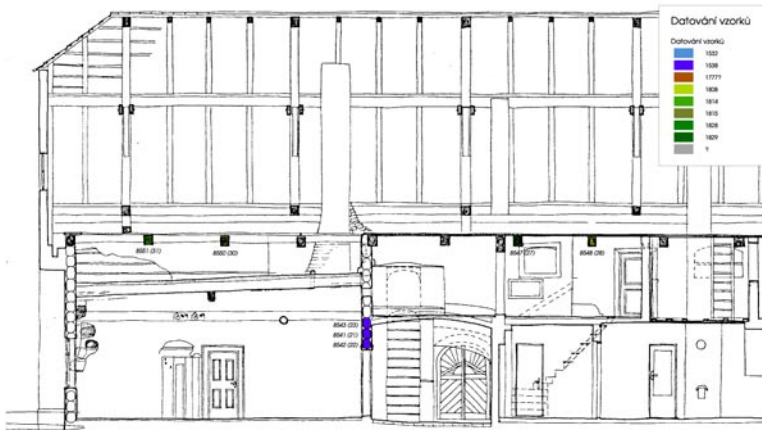
Dendrochronologie - řez DD
