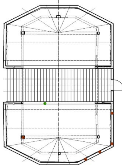
Trstěnice čp. 41 (SY) - polygonální stodola dendrochronologicky datovaná 1663 (mlat 1809) * 128 - 131 - interier * 132 - půdorys a příčný řez * 133 - detail konstrukce mlatu * 134 - celkový pohled z humna * 135 - východní pohled (stav 1988) * 136 - připojená kolna
