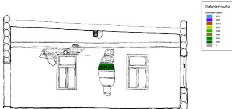
Dendrochronologie - řez BB
