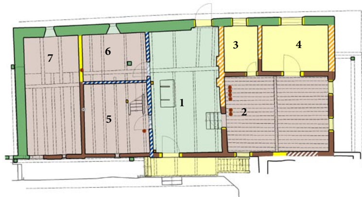
1 - síň * 2 - obytná místnost (1664) * 3 - spízní komora * 4 - světnička * 5 / 6 - komory * 7 - chlév
