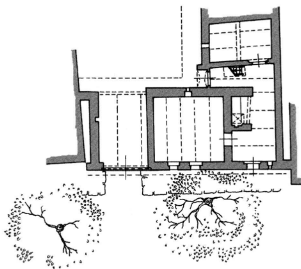
Obr. 2. Velká nad Veličkou (okr. Hodonín), dům čp. 117; půdorys přízemí přízemního domu s rohovou síní podle J. Vajdiše. – Abb. 2. Velká nad Veličkou (Bez. Hodonín), KNr. 117; Grundriss des erdgeschossigen Hauses mit Eckhalle, nach J. Vajdiš.
