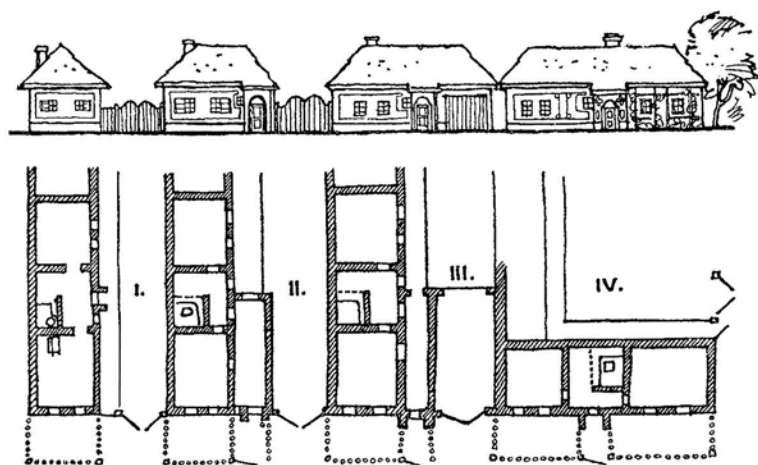
Obr. 1. Tvrdonice (okr. Břeclav); vývoj orientace domu usedlosti podle J. Kouly (Koula 1894). – Abb. 1. Tvrdonice (Bez. Břeclav); Entwicklung der Orientierung eines Guts-hauses nach J. Koula (Koula 1894).
